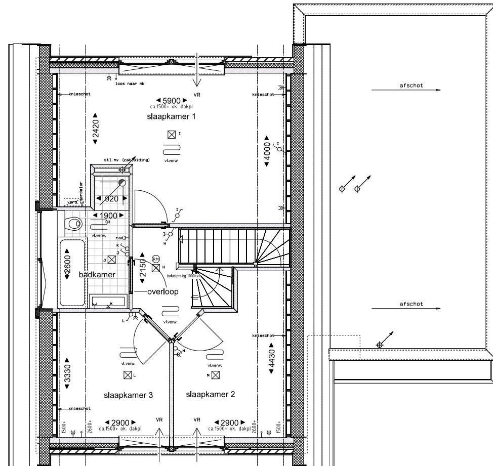
1e Verdieping
