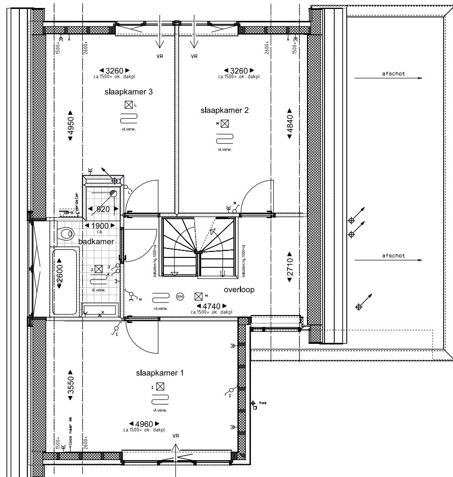
1e Verdieping
