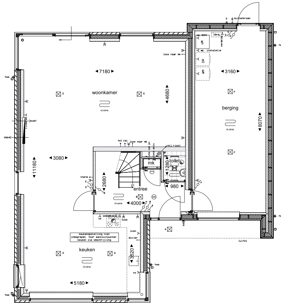
Begane grond
