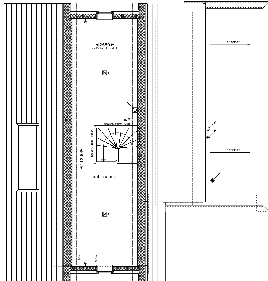
2e Verdieping
